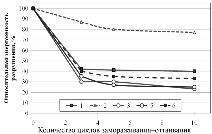
Рис. 2. Относительная энергоёмкость разрушения горных пород в зависимости от циклов замораживания–оттаивания (5 %-й солевой раствор). Усл.обозначения приведены на рис. 1
