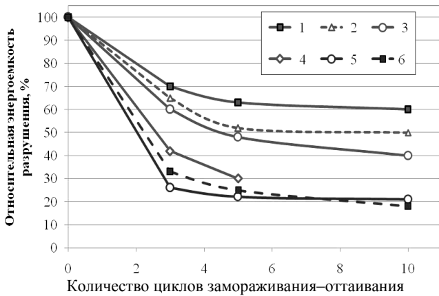
Рис. 1. Относительная энергоёмкость разрушения горных пород в зависимости от циклов замораживания–оттаивания (водная среда):
