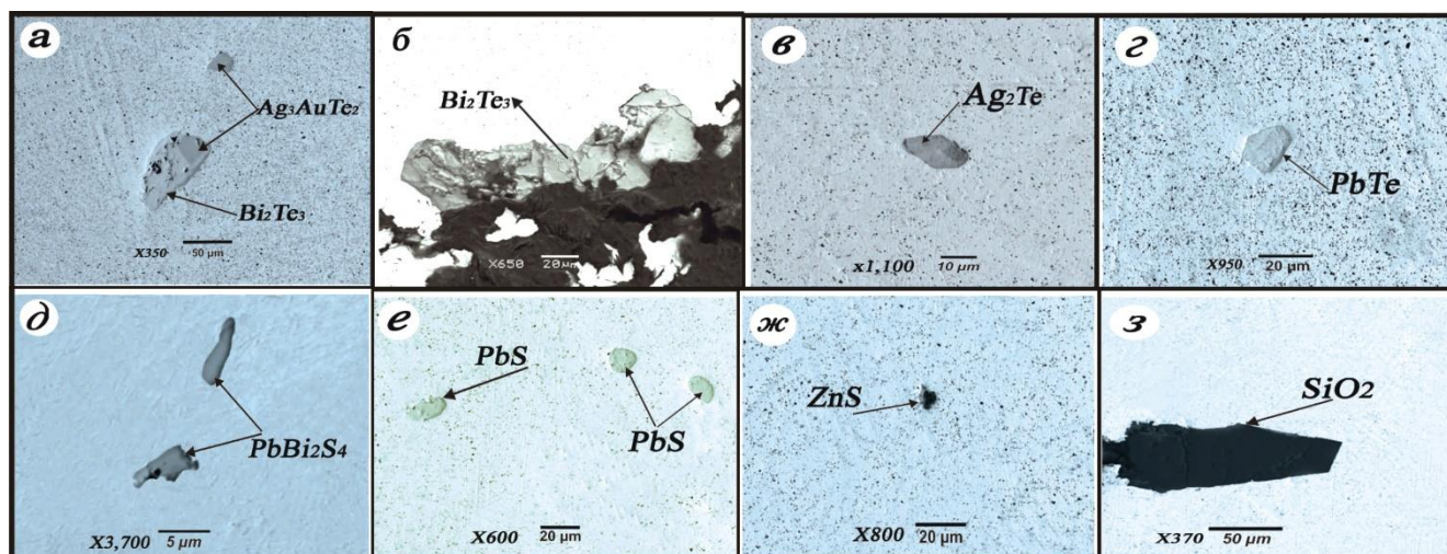
Рис. 3. Микровключения в россыпном золоте Хатырхайского узла: а – двухфазное идиоморфное обособление теллуrowисмутита \text{Bi}_2\text{Te}_3 (серый), петцита \text{Ag}_3\text{AuTe}_2 (темно-серый) в самородном золоте; б – обособление теллуrowисмутита \text{Bi}_2\text{Te}_3 на границе срастания золота с гематитом (серое); в – идиоморфное обособление гессита \text{Ag}_2\text{Te} (темно-серые пятна с содержанием \text{Hg} 34 %); г – включение алтаита \text{PbTe} в самородном золоте; д – идиоморфные включения сульфowисмутита свинца \text{PbBi}_2\text{S}_4 в самородном золоте; е – обособления галенита \text{PbS} в самородном золоте; ж – включение сфалерита \text{ZnS} в самородном золоте; з – крупное угловатое включение кварца \text{SiO}_2 в самородном золоте
