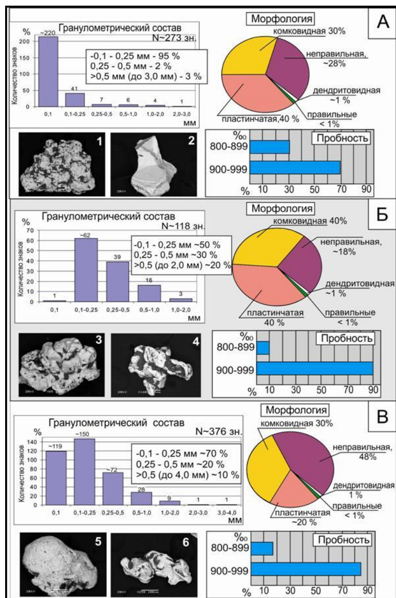
Рис. 2. Морфология, гранулометрический состав и пробность россыпного золота по ручьям: А – Таяхтах; Б – Горелый; В – Крутой. Форма золотин: 1 – пластинчатая с мелкоямчатой поверхностью и пленками гидроокислов железа; 2 – с ограниченными кристаллическими выступами; 3 – комковидная с бугорчатой поверхностью; 4 – гемиидиоморфная с ямчатой поверхностью; 5 – комковидная с шагреновой поверхностью; 6 – дендритовидная
